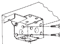
Jamb Mount FIG. 6
